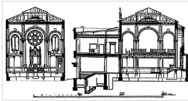
Plans de la synagogue de la rue Kageneck, du bain rituel et des salles de classe. Coupe transversale et en longueur - Strassburg und seine Bauten , 1884, p.399
